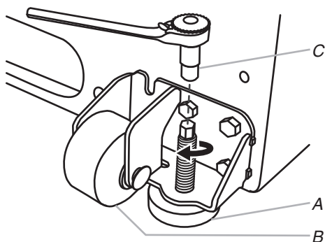
A. Pata con freno B. Rodillo frontal C. Llave de hexagonal de 1/4"
