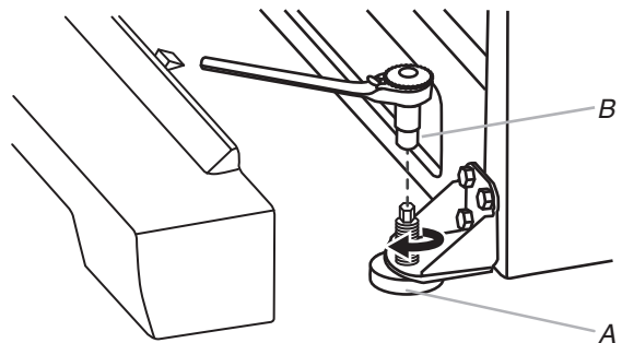
A. Pata con freno B. Llave de hexagonal en L de 1/4"
